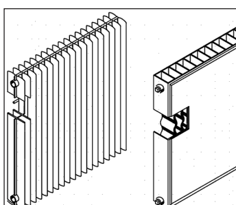
61 Faltradiatoren
