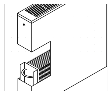
73 Konvektoren Fertigverkleidung
