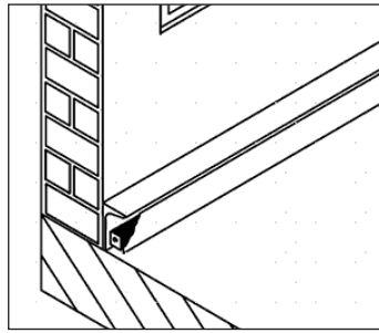
76 Konvektoren Fußleisteneinbau
