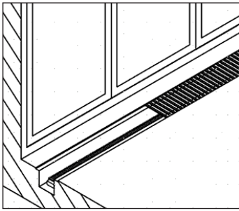
74 Konvektoren Unterflohreinbau
