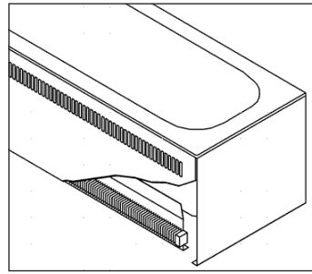
75 Konvektoren Badewannenverkleidung
