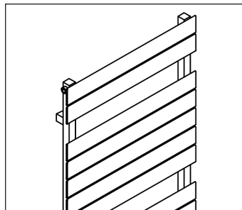
33 Flachprofil-HK Sonderform
